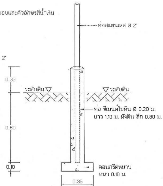
รูปตัด มาตราส่วน 1 : 15
